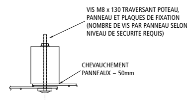
SECTION POTEAU INTERMEDIAIRE
